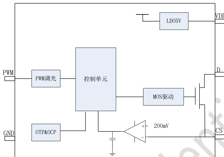
图 7.1 结构框图
