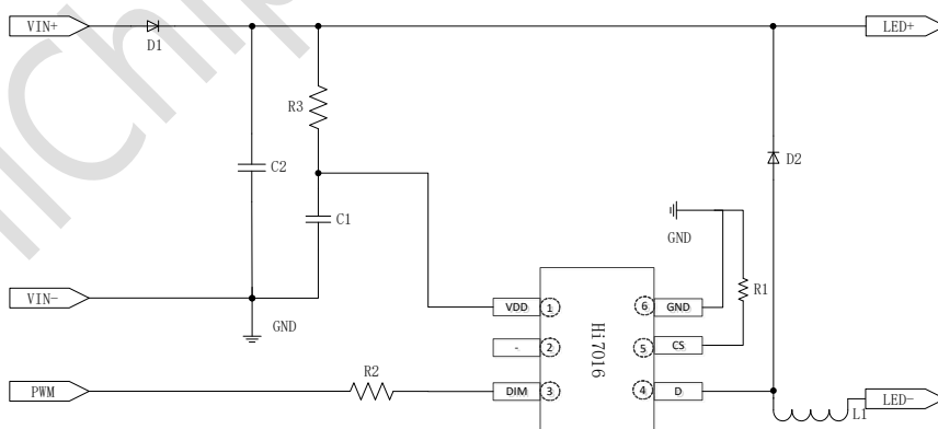
图 4.1 Hi7016 应用电路
