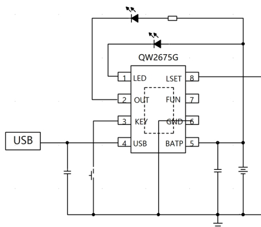
QW2675G 典型应用电路
