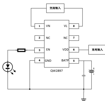
图一 QW2897 典型应用电路
