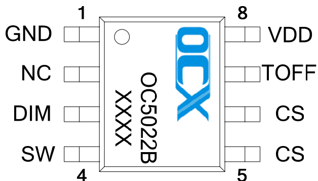
ESOP8
