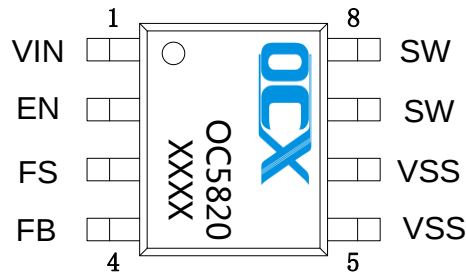
SOP8
