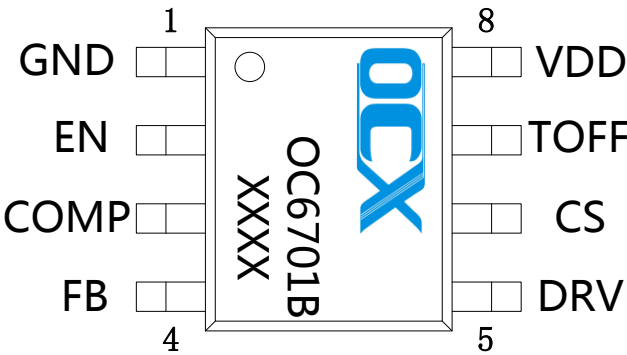
SOP8
