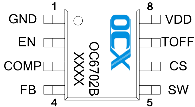
ESOP8
