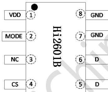
图 5.1 Hi2601B 引脚图
