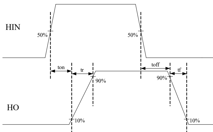
图 2 高侧端输出 HO 开关时间波形图
