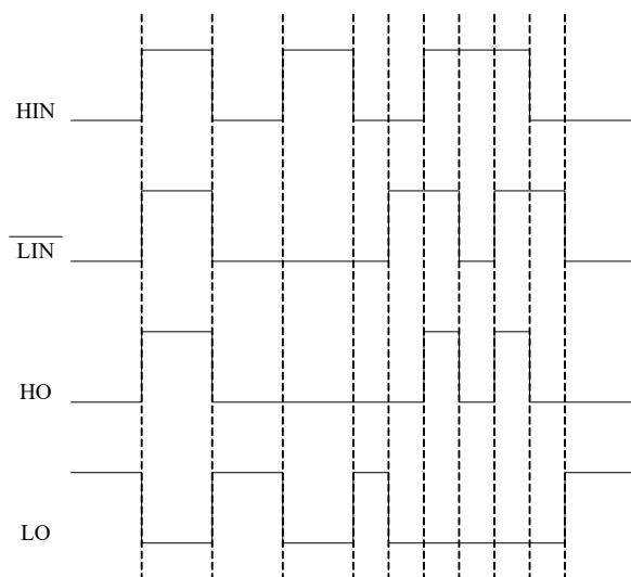
图 4 典型输入输出时序
