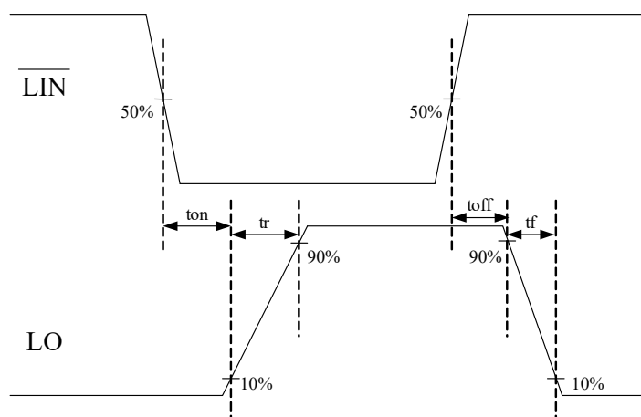
图 1 低侧端输出 LO 开关时间波形图
