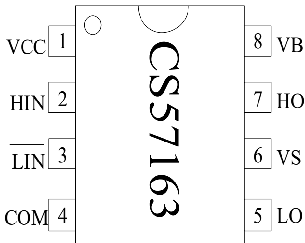
引脚排列图
