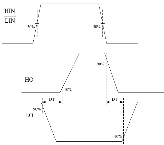
图 3 死区时间波形图
