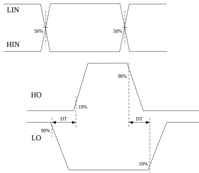
图 2 死区时间波形图
