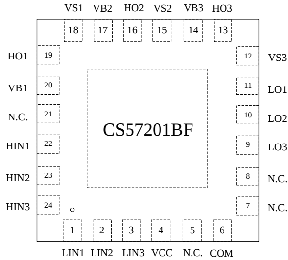
QFN24 引脚排列图
