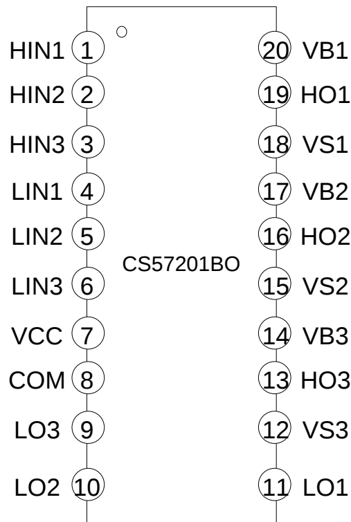
TSSOP20 引脚排列图
