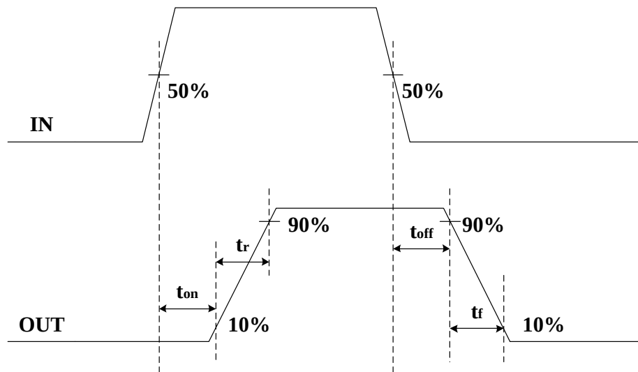
图 1 开关时间波形图
