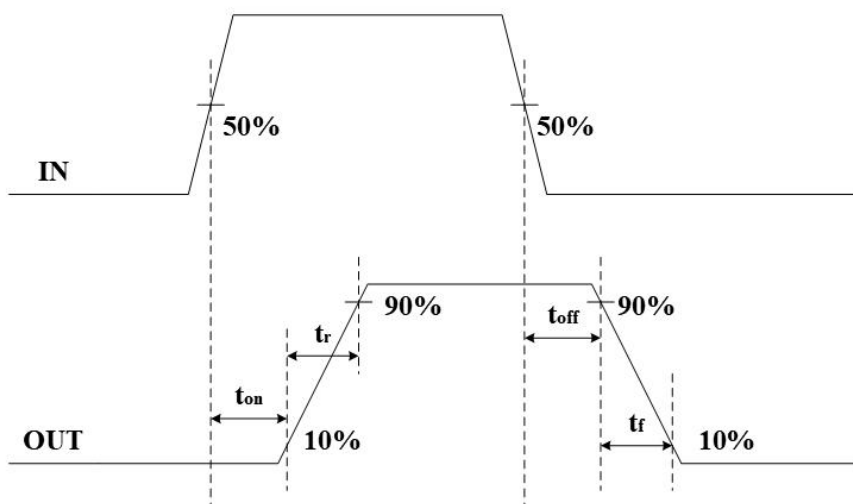
图 1 开关时间波形图
