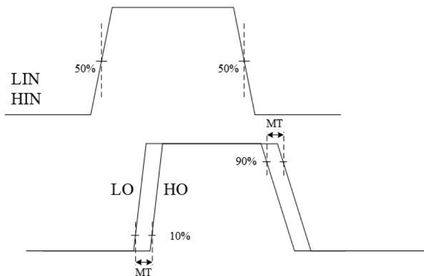
图 3 延时匹配 MT 波形图
