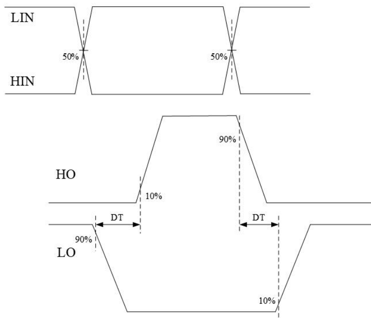
图 2 死区时间波形图
