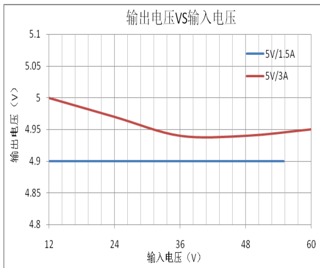
(2) 输出 5V/12V, 1.5A/3A 输出与输入电压特性曲线
