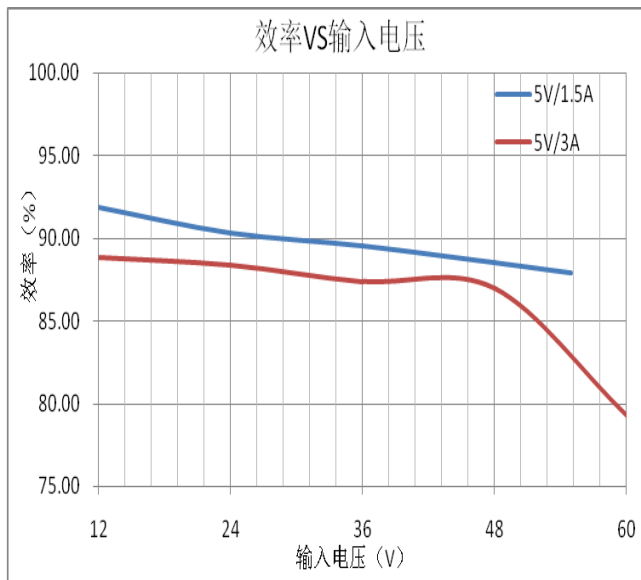
(2) 输出 5V/12V, 1.5A/3A 输出与输入电压特性曲线
