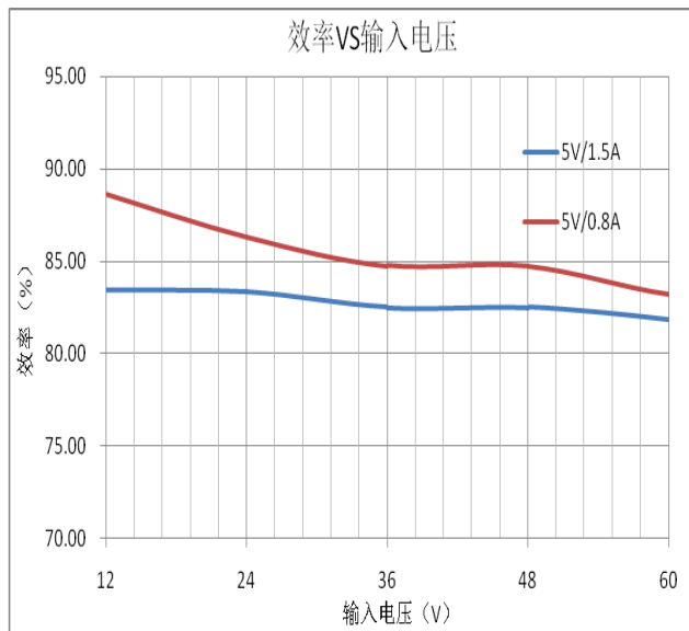
(2) 输出 5V/12V, 0.8A/1.5A 输出与输入电压特性曲线
