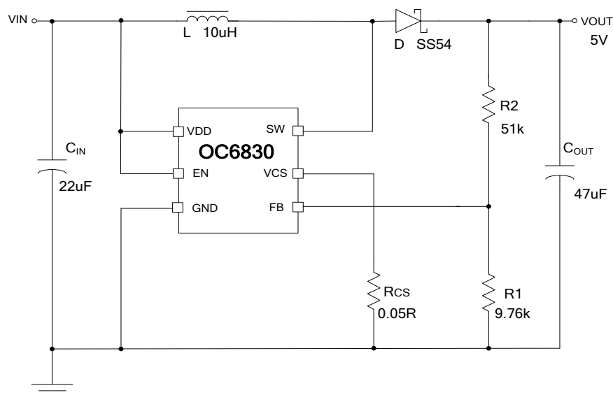
OC6830 典型应用电路图
