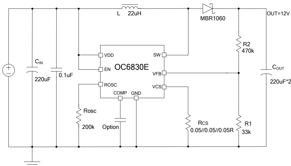
OC6830E 典型升压应用电路图
